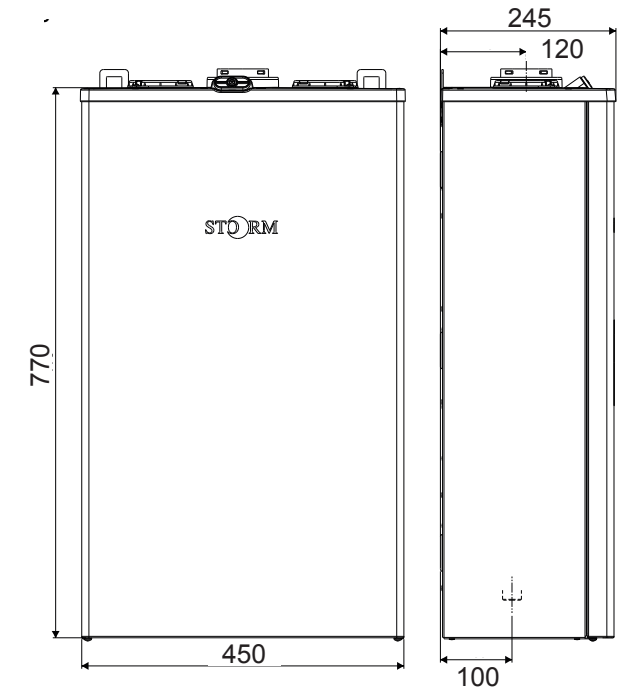
Fig.1 - Vista frontale / Vista laterale
