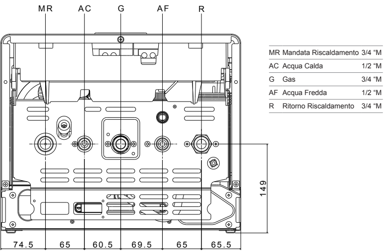
Fig.2 - Vista dal basso - schema connessioni idrauliche (tipo DIN)
