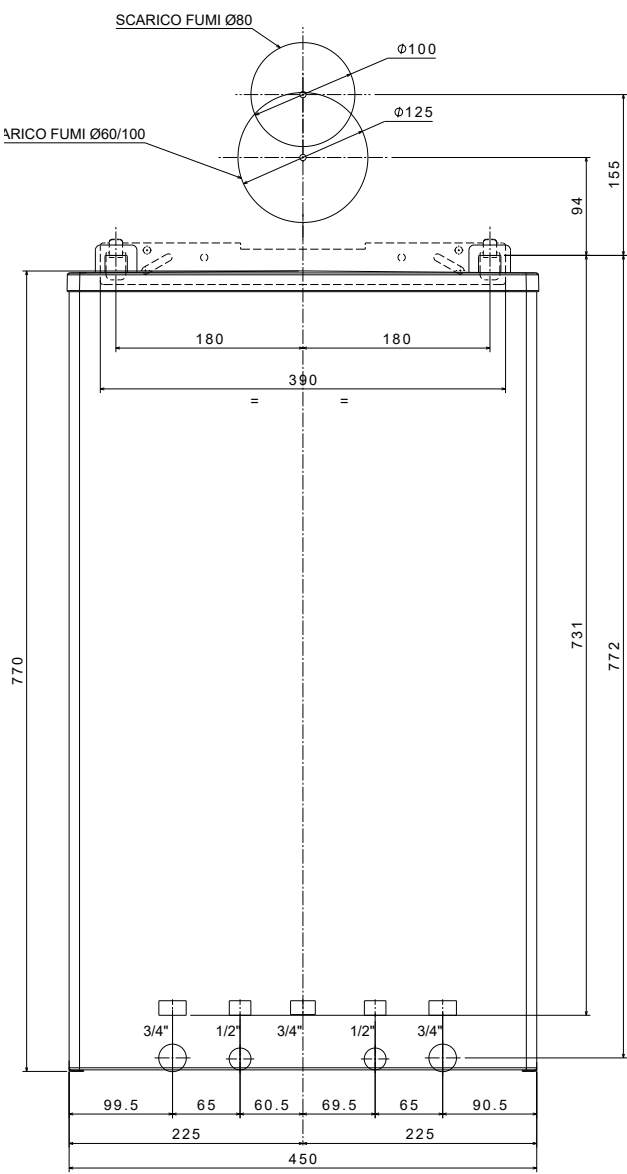
Fig.4 - Fissaggio della caldaia a muro e allacciamenti idraulici
