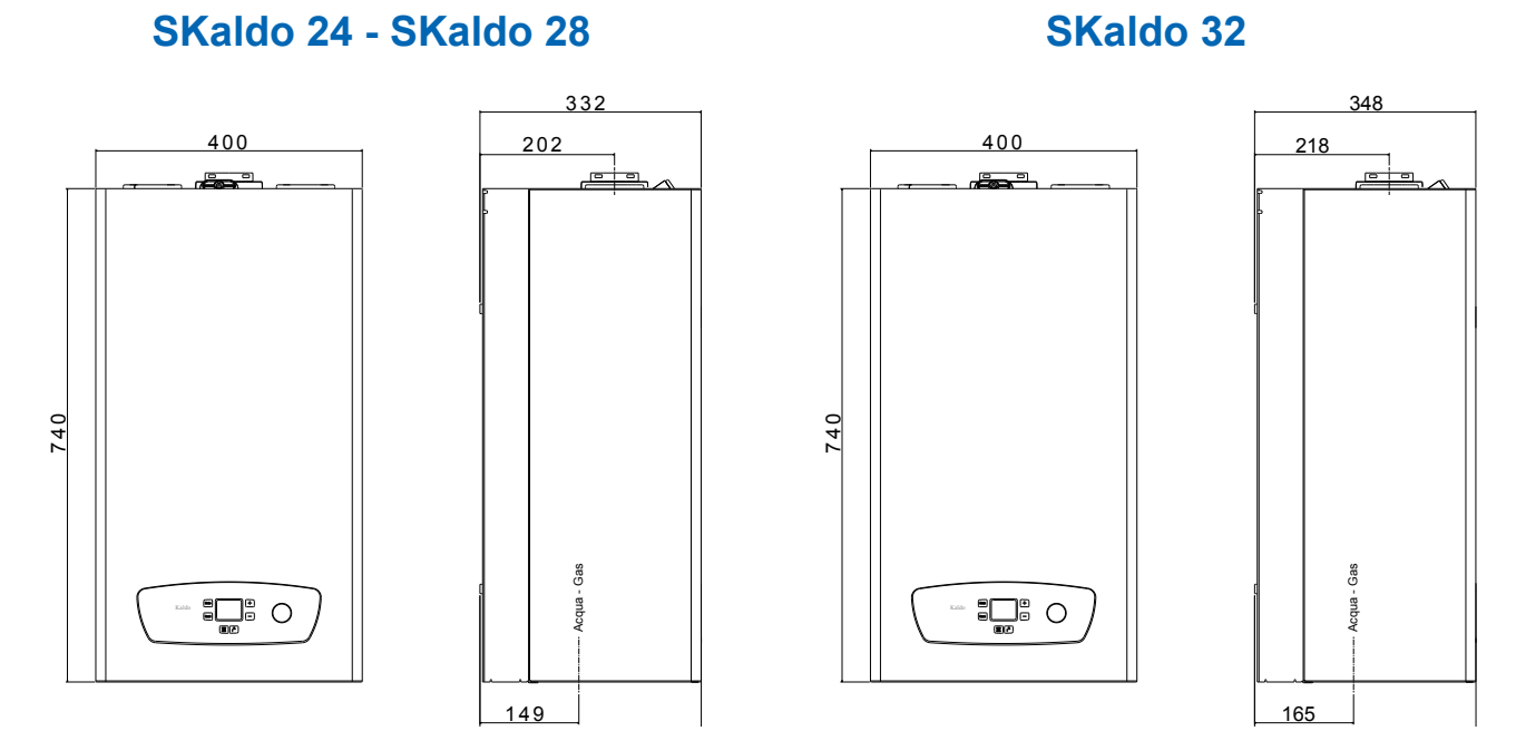
Fig.1 - Vista frontale / Vista laterale
