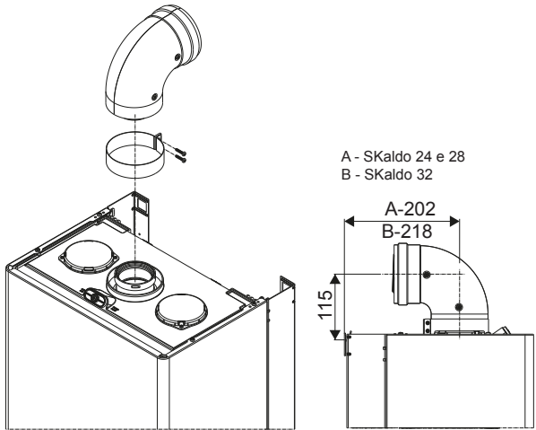
Condotti coassiali ø 60/100
