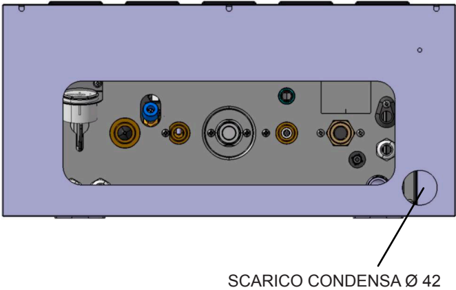
Fig.2 - Vista dal basso - spazio per connessioni
