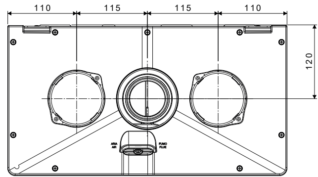
Fig.2 - Vista dall'alto - Collegamento condotti aspirazione e scarico fumi
