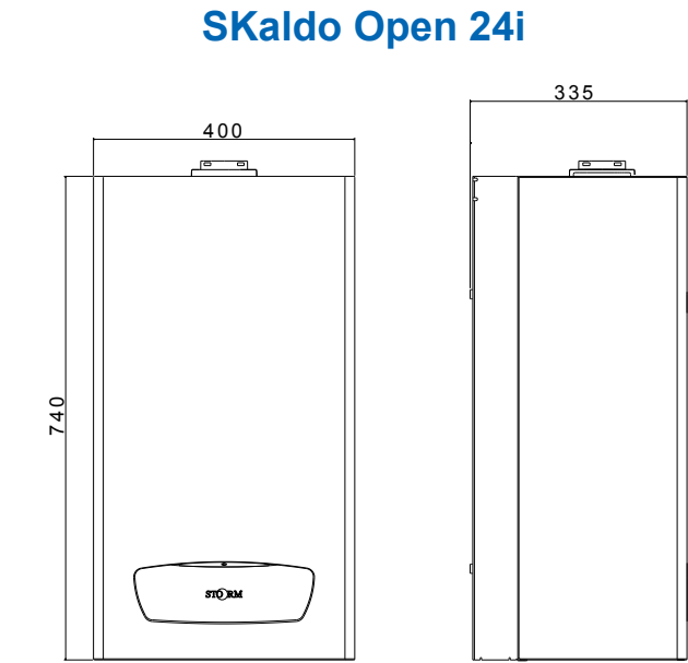
Fig.1 - Vista frontale / Vista laterale
