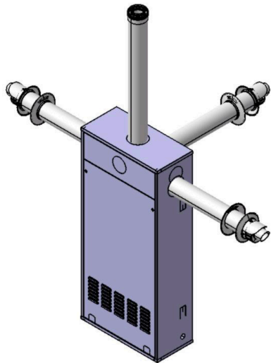
Fig.3 - Soluzioni per sistema di scarico ø60/100
