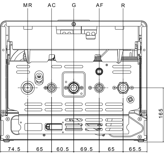
Fig.5 - Vista dal basso - schema connessioni idrauliche (tipo DIN)
