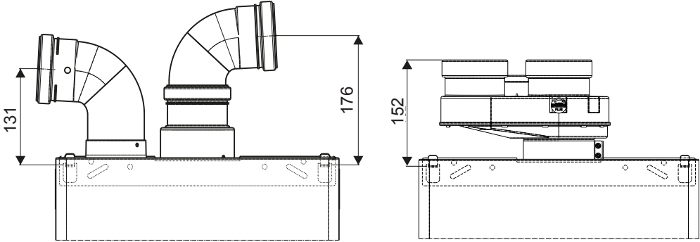
Condotti sdoppiati ø 50 / ø 60 / ø 80
