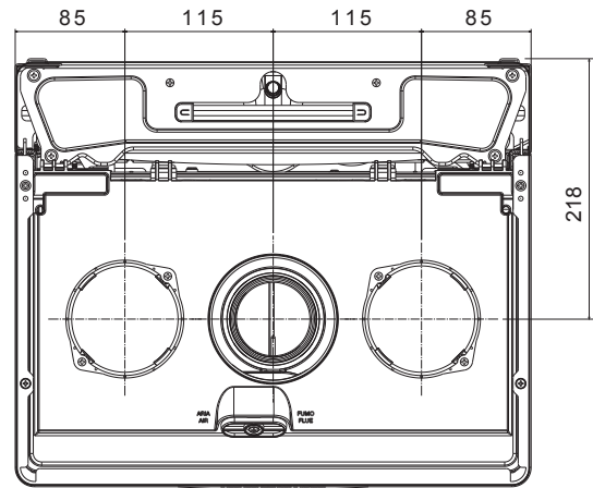
Fig.6 - Vista dall'alto - schema connessioni scarico fumi - aspirazione aria comburente
