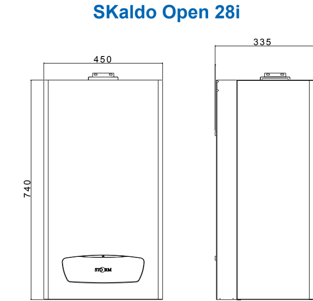
Fig.2 - Vista frontale / Vista laterale
