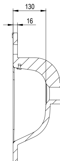
SEZIONE A-A
