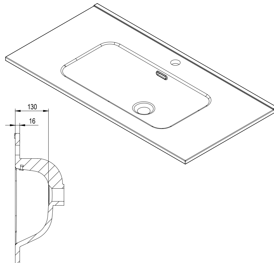
SEZIONE A-A
