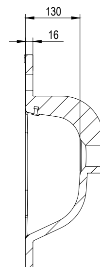
SEZIONE A-A
