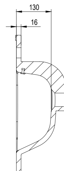
SEZIONE A-A
