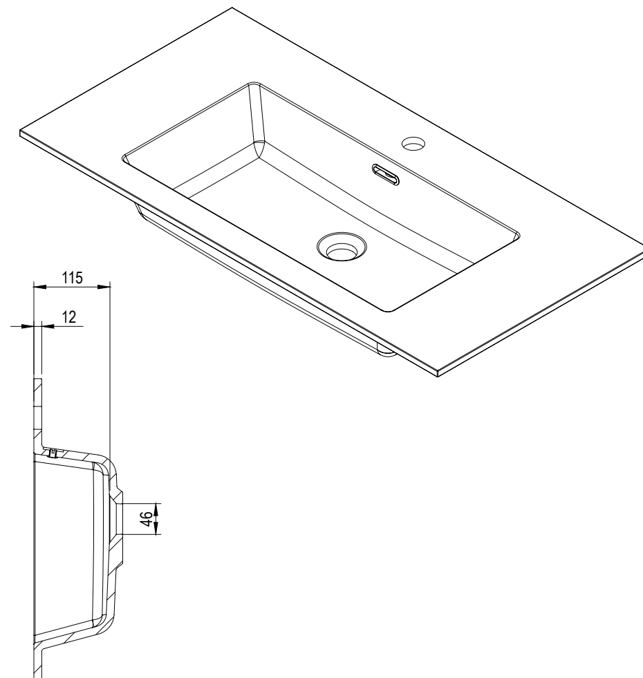
SEZIONE A-A
