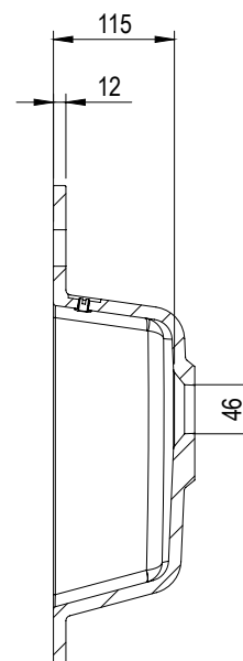
SEZIONE A-A
