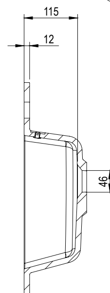
SEZIONE A-A
