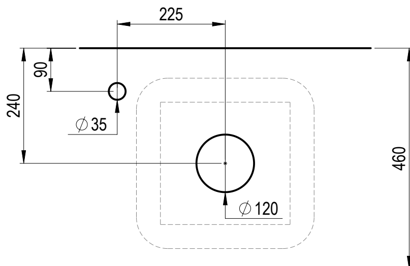
RUBINETTO DESTRA/SINISTRA
