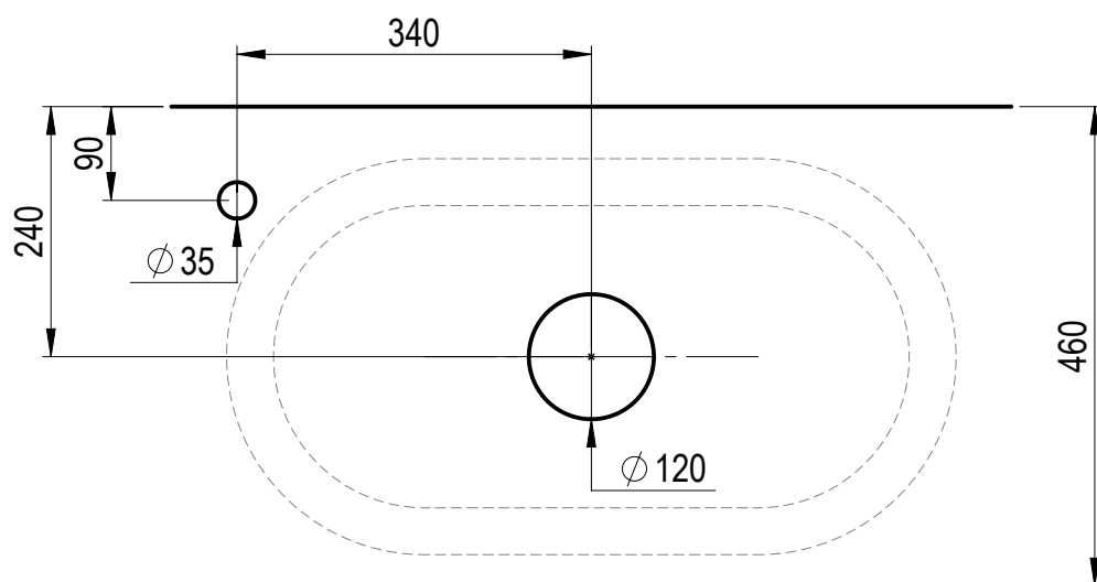
RUBINETTO DESTRA/SINISTRA
