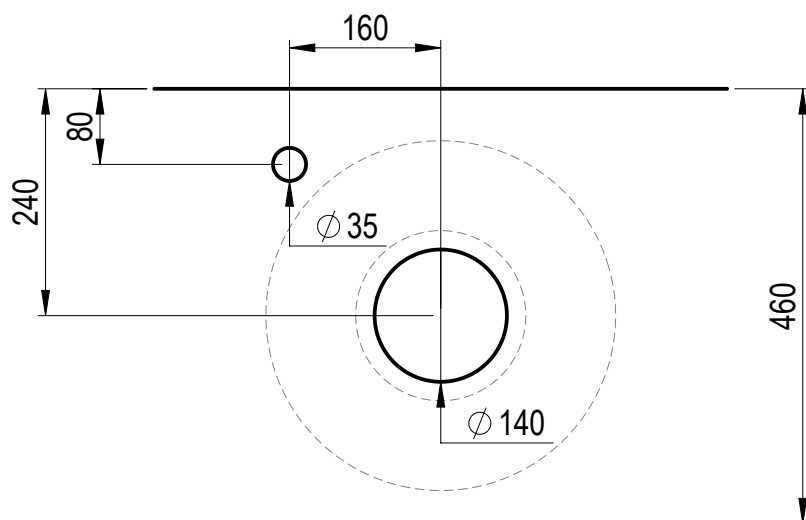
RUBINETTO DESTRA/SINISTRA
