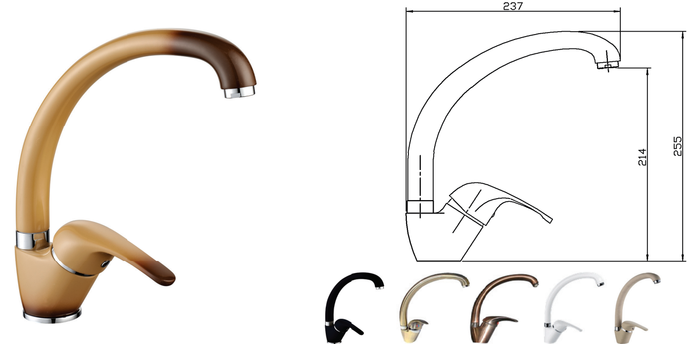
Miscelatore monocomando per lavello Single lever sink mixer
