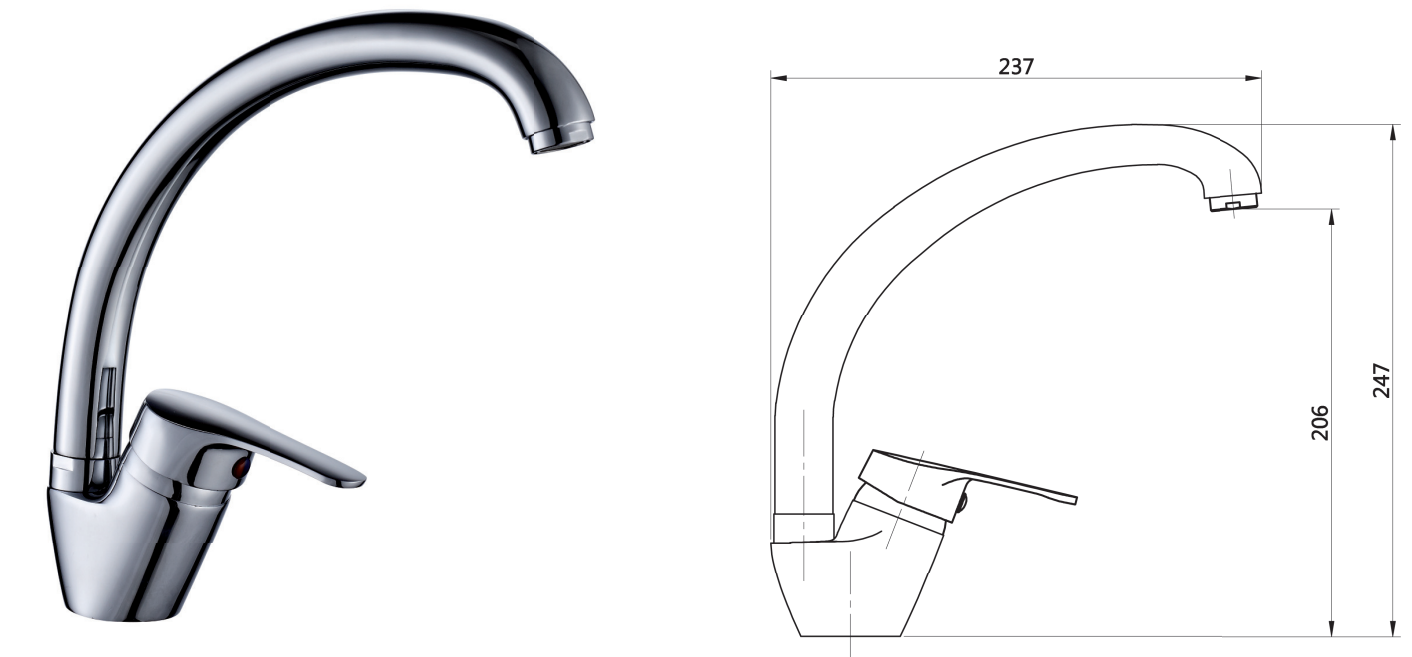
Cartuccia ø 40 Cartridge ø 40
