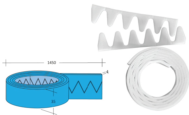
Protezione antiurto e acustica autoadesiva a zig-zag per tutte le tipologie di sanitari - spessore 4 mm.
