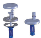
Cerniere C4501H Topf. da alto Fissaggio EasyFix a espansione disco scanalato Acciaio inox e base nylon.
