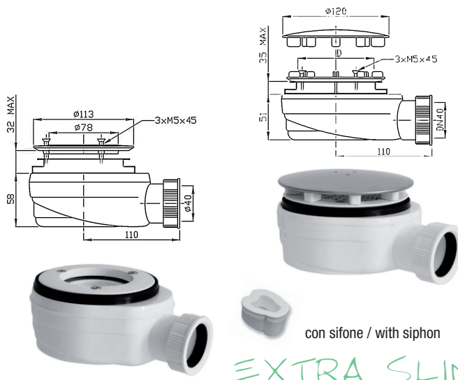
Scarico doccia EXTRA SLIM 90 x 40 altezza 51 mm. uscita acqua 52 l/min.
