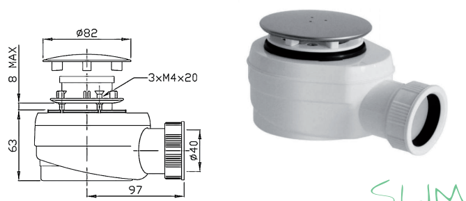
Scarico doccia SLIM 50 x 40 altezza 62 mm. uscita acqua 52 l/min.
