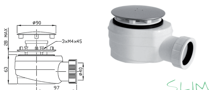
Scarico doccia SLIM 60 x 40 altezza 62 mm. uscita acqua 52 l/min.
