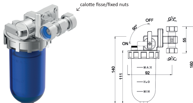
Dosatori proporzionali di polifosfato attacco laterale con calotte fisse Proportional polyphosphate feeders side connection and fixed nuts
