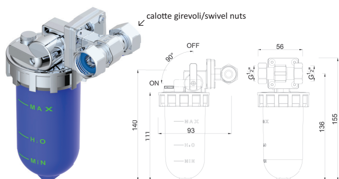
Dosatori proporzionali di polifosfato attacco laterale con calotte girevoli Proportional polyphosphate feeders side connection and swivel nuts
