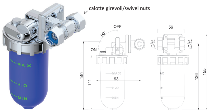
Dosatori proporzionali di polifosfato attacco laterale con calotte girevoli Proportional polyphosphate feeders side connection and swivel nuts cod. pz. x conf. euro cad. 1484DOSP40 1/2" FF 12 55,700
